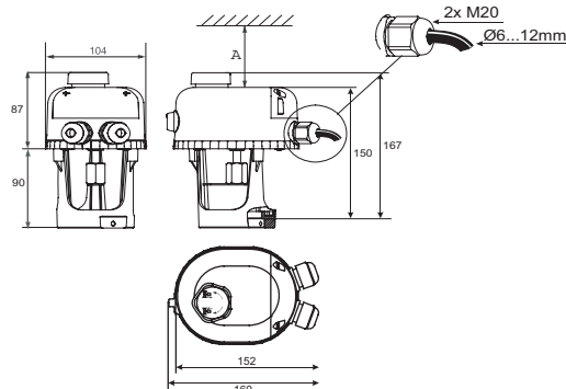
A 25 mm VA-770x 电动执行器, 无手动操作功能 A 80 mm VA-774x 电动执行器, 带手动操作功能
